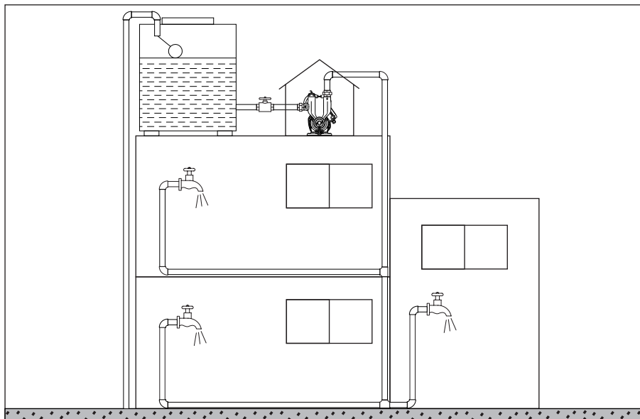
Tanque superior de água
